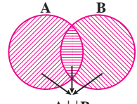
A \cup B اجتماع دو مجموعه
