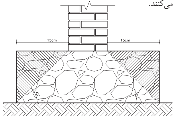
شکل ۱-۳۴ پی سنگی با زاویه پخش بار در پی های سنگی ۴۵ درجه است.
