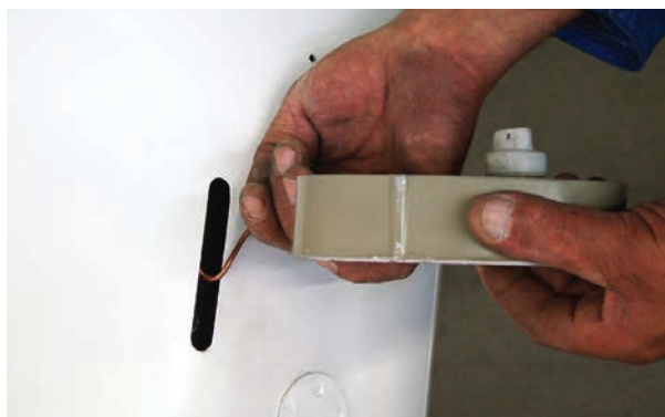
شکل ۵۶-۱- ب - قرارگیری صحیح بالب ترموستات در محل خود
