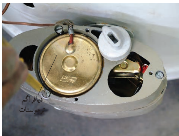
شکل ۵۵-۱- ب - دیافراگم ترموستات
