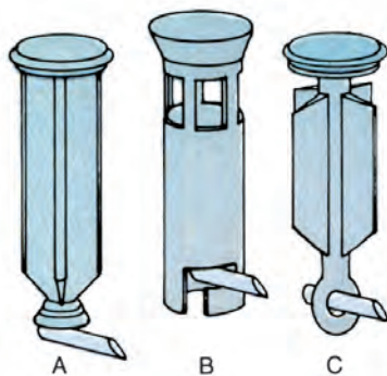
شکل ۴-۲- جزئیات ارتباط ضامن با سرپوش فلزی زیراب
