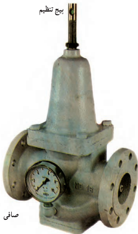
شکل ۲-۱۰۲- شیر فشار شکن
