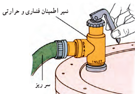
شکل ۱۰۹-۲ شیر اطمینان فشاری - حرارتی
