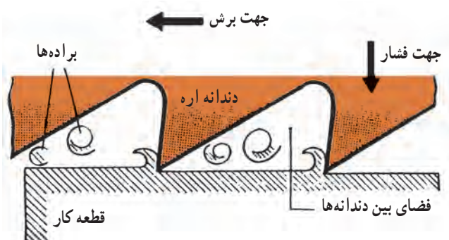
شکل ۱-۱- دندانه‌ی تیغه‌اره
