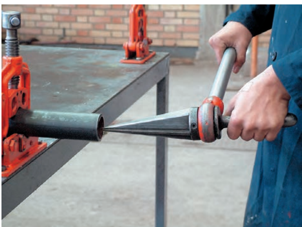
شکل ۱۱-۲- مرحله‌ی اول برقوقاری
