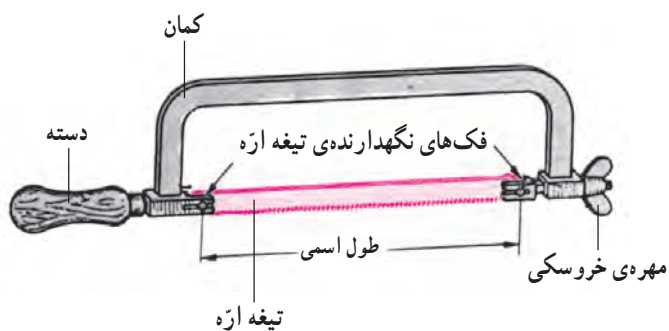
شکل ۱-۴- اجزای کمان اژه
