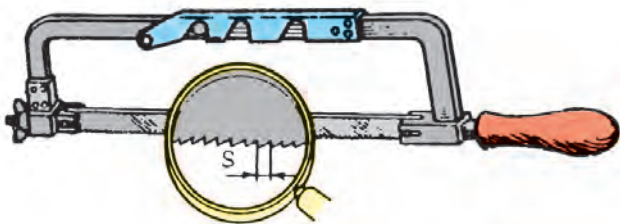
شکل ۱-۱۵ - گام دندانه‌ی تیغه‌ی اژه
