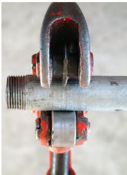
شکل ۹۶-۵- استفاده‌ی غلط از لوله‌بُر با تیغه‌ی شکسته
