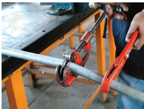
شکل ۱۱۷-۵- بریده شدن لوله و خاتمه‌ی کار
