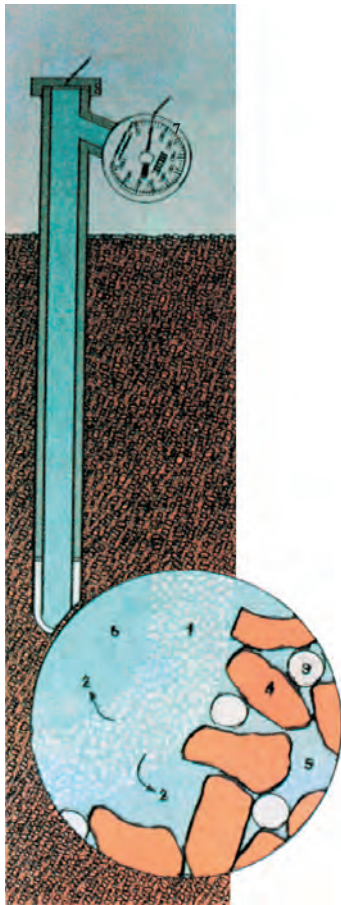
شکل ۱۸-۱- تانسئومتر و نحوه قرار گرفتن آن در خاک
