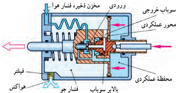
شکل ۳۱-۱- بوستر ترمز نیوماتیکی
