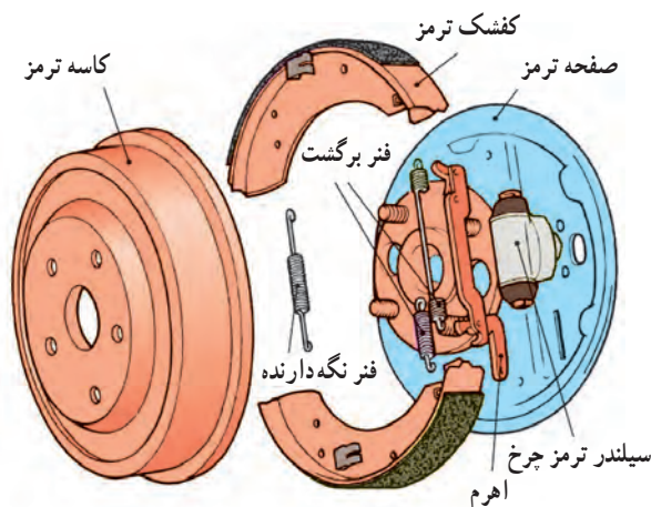
شکل ۱-۳۵- ترمز کفشکی
