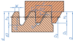
رزوه‌های اراده‌ای متریک طبق DIN 513 (1985-04)
