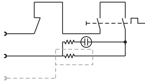
شکل ۱-۲۳ نقشه ی مدار الکتریکی کتری برقی قسمتی از چای ساز
