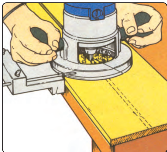
شکل ۵۶-۲ ایجاد شیار کنشکاف به کمک گونیا و ماشین اورفرز دستی برقی
