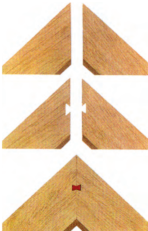
شکل ۱۱۴-۲ مراحل اجرایی اتصال دم چلچله گوشه‌ای قاب
