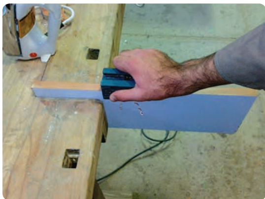
شکل ۱۵۶-۲ رنده پرداخت لبه نوار روکش لبه چسبان
