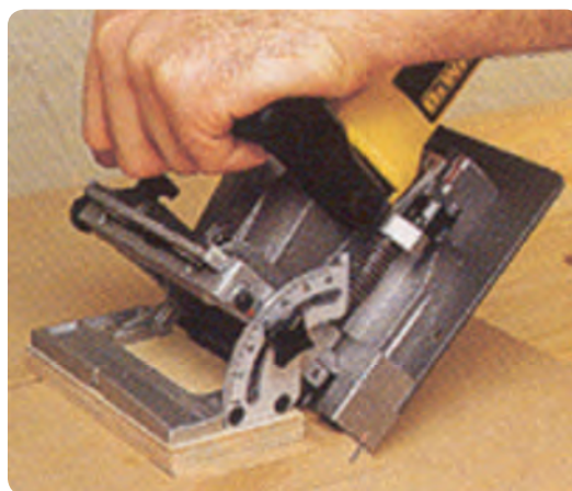
شکل ۲-۹۰ شیارزنی با زاویه ۴۵ درجه
