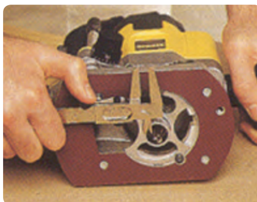
شکل ۶۸-۲ اندازه‌گیری قطر شفت فرز
