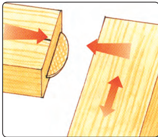
شکل ۸۴-۲ نحوه جازدن اتصال بیسکویتي
