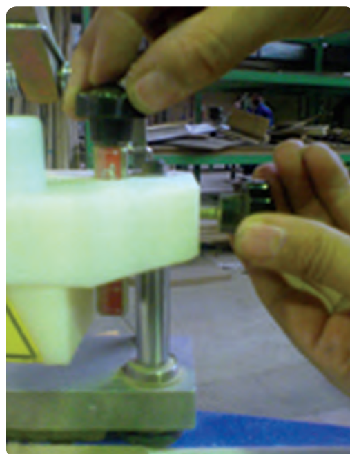
شکل ۱۱۳-۲ تنظیم عمق فرز جهت اتصال
