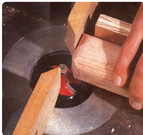
شکل ۲-۶۳ فرز زدن کله چوب با اورفرز دستی برقی
