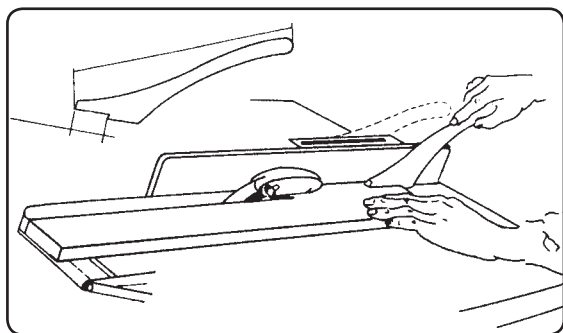
شکل ۳-۱۶ شابلون حفاظتی هدایت چوب از کناره‌اره گرد
