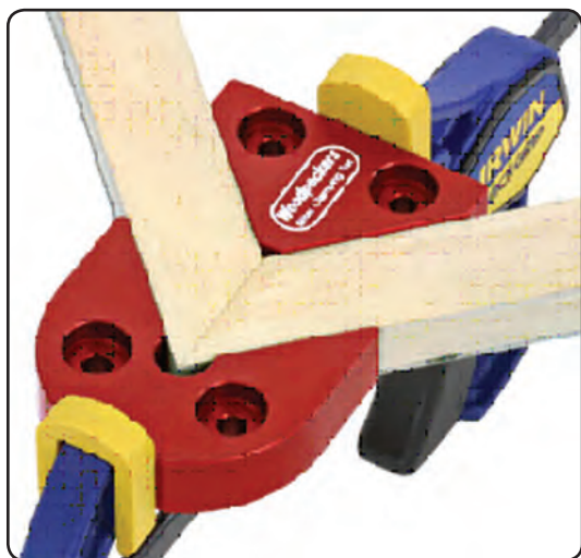
شکل ۳-۳۳ فیکسچر جهت مونتاژ قاب به حالت افقی
