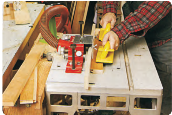
شکل ۳-۳۰ شابلون کمکی و حفاظتی جهت فرز کردن قطعات کوچک
