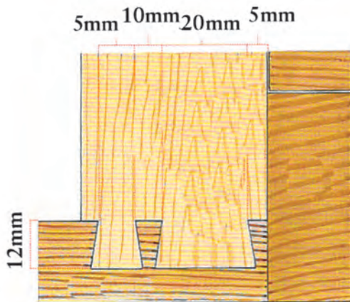
شکل ۵۷ - ۸ فایل اتصال دم‌چلچله در قید پایین پایه
