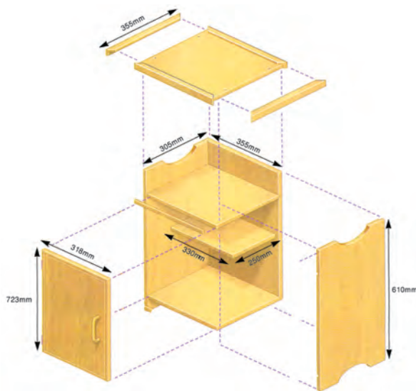
شکل ۸-۳۵ نقشه مونتاژ قطعات کابینت
