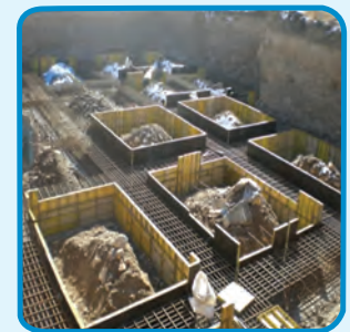
شکل ۳-۳۱- قالب فایبرگلاس برای اجرای پی
