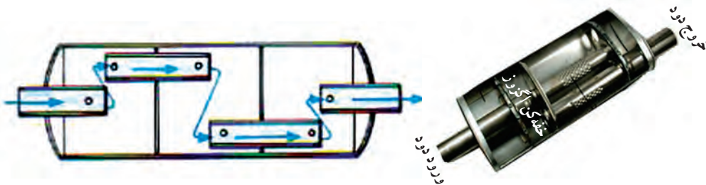
شکل ۲۵-۵- خفه کن معکوس
