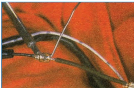
شکل ۶۴-۶- نحوه لحیم کاری سیم‌ها
