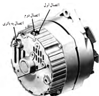
شکل ۲۶-۶- آلترناتور
