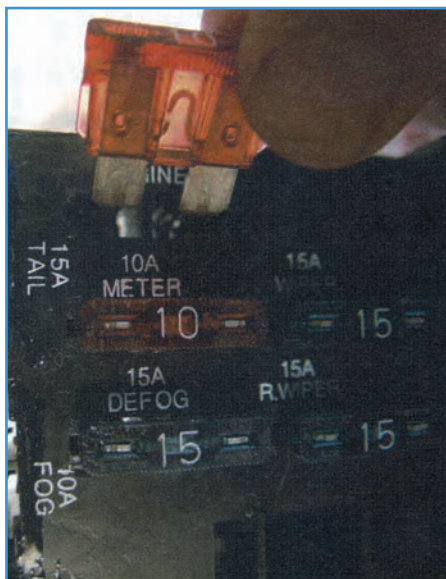
شکل ۶۹-۶- جازدن فیوز در محل آن
