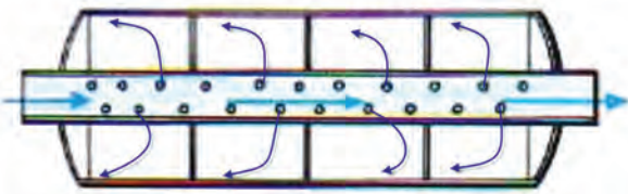
شکل ۲۴-۵- صدا خفه کن یکسره
