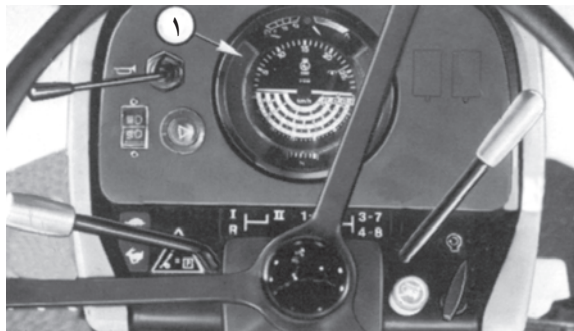
۱ - دورسنج
