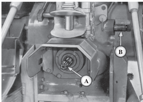
A - محور انتقال نیرو ۶ شیاره B - محور انتقال نیرو، یدکی ۲۱ شیاره
