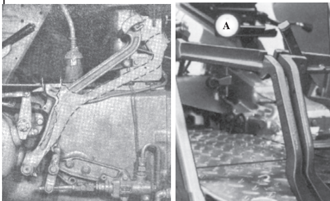
— پدال ترمز
