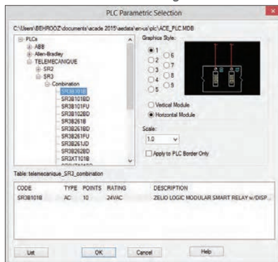
شکل ۴۳- رله قابل برنامه‌ریزی
