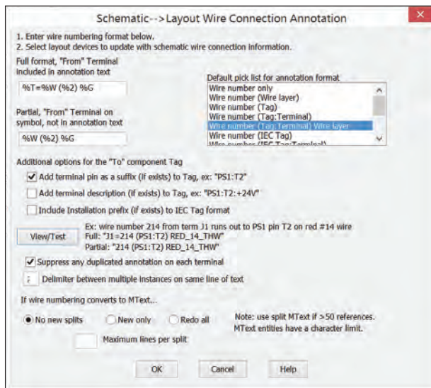
شکل ۵۵- دستور حاشیه‌نویسی سیم‌ها
