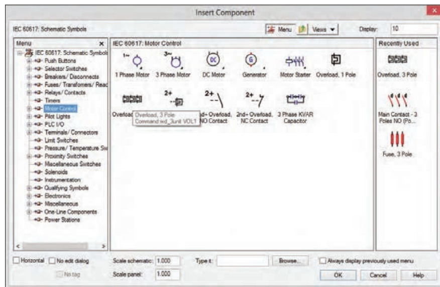
شکل ۱۴- انتخاب رله اضافه بار بی متال
