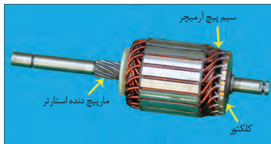
شکل ۳۷- آرمیچر استارت‌تر
