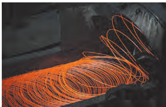
شکل ۴ ▲ نورد گرم میل گرد
