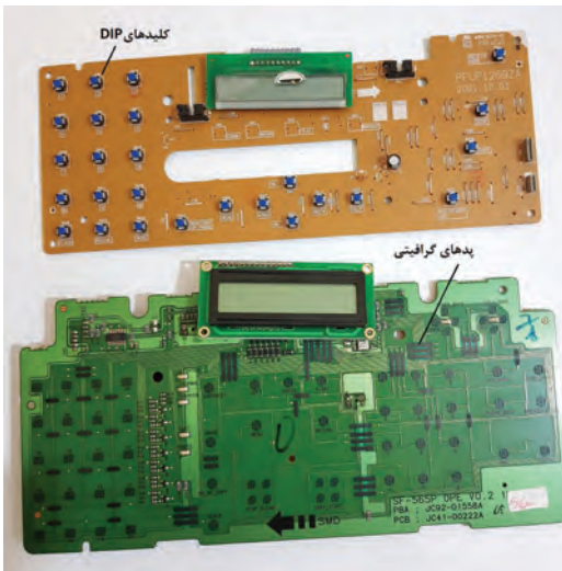
شکل ۳-۴۱- دونمونه پنل دستگاه چهارکاره
