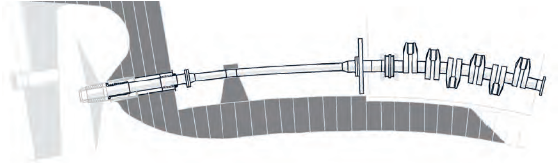
شکل ۱۴- خمش محور در اثر بارهای بیرونی که جهت درک بهتر به شکل اغراق آمیز نشان داده شده است
