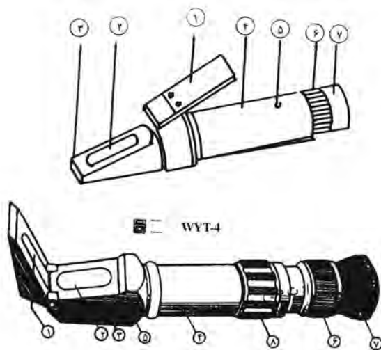
شکل ۳- رفراکتومترهای دستی
