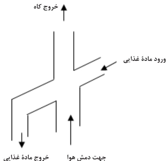
شکل ۱- اصول کار آسیپراتور
