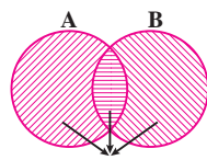
A \cup B اجتماع دو مجموعه
