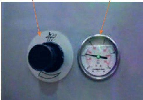
شکل ۶۷- تنظیمات فشار پرس رول طرف اپراتور
