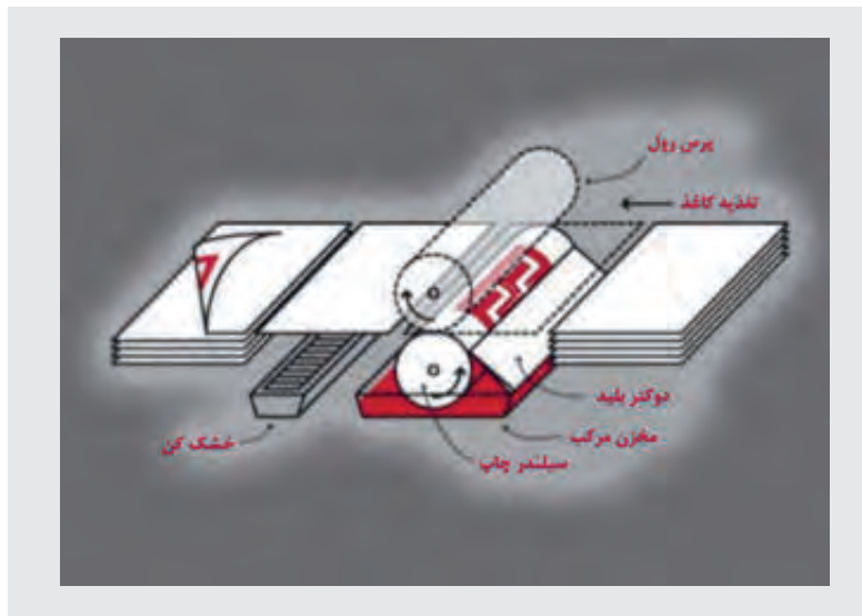
شکل ۳۹- نقشه شماتیک دستگاه تغذیه ورقی
