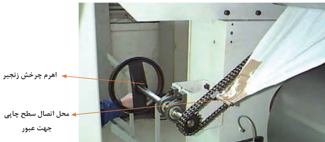
شکل ۵۸- زنجیر گیره‌ای
