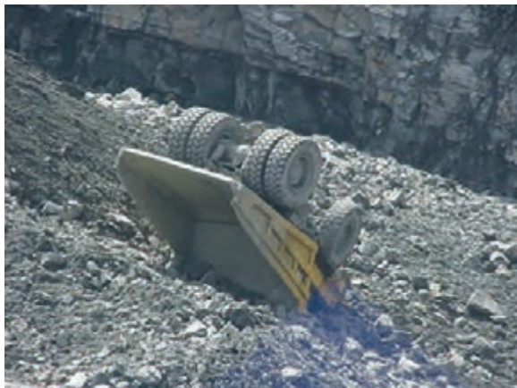
سقوط یک دامپتراک به دلیل عدم وجود دیواره اطمینان (Berm)
