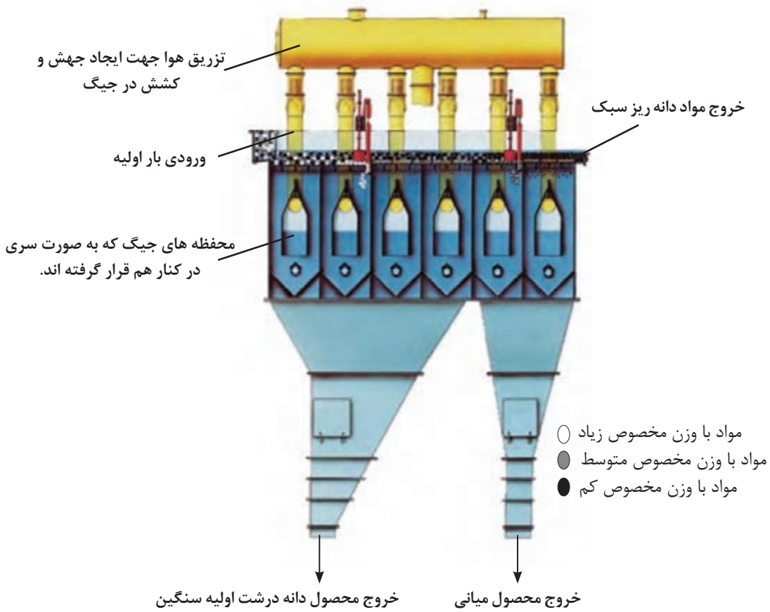
شکل ۵- شماتیک جیگ باتاک
