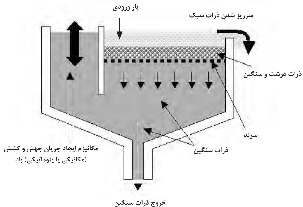
شکل ۱- مکانیزم جدایش ثقلی در جیگ
