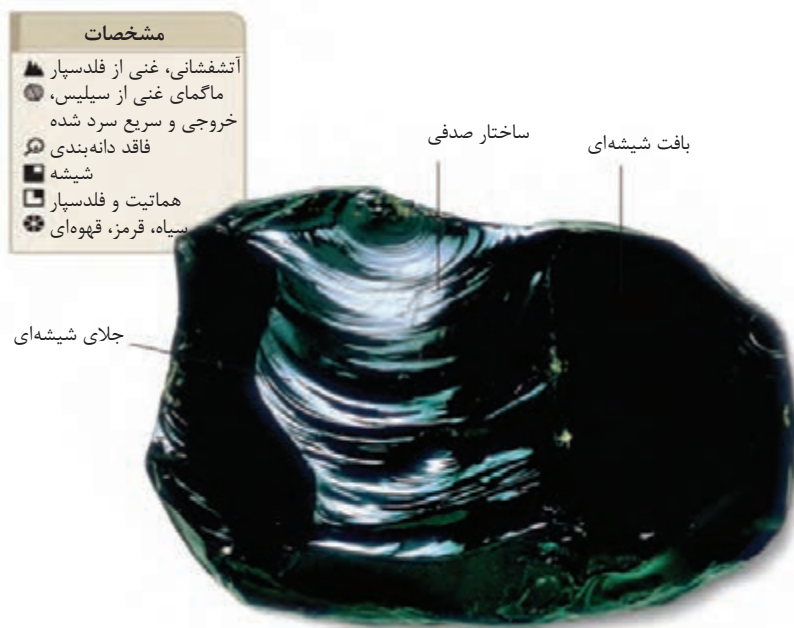
شکل ۲-۲۶ - ابسیدین
