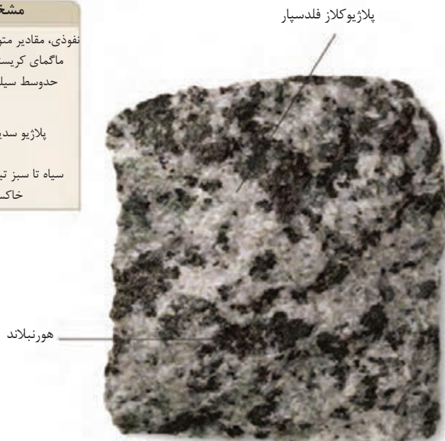
شکل ۲-۲۲- دیوریت
