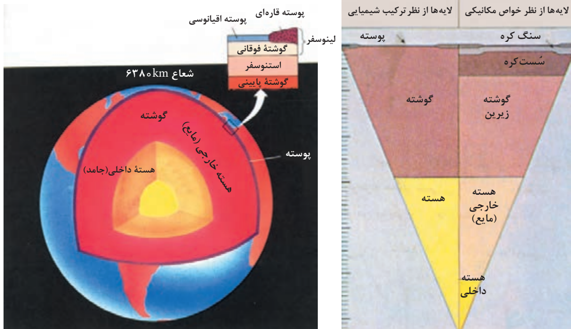
شکل ۲-۶- لایه‌های زمین (۴)
