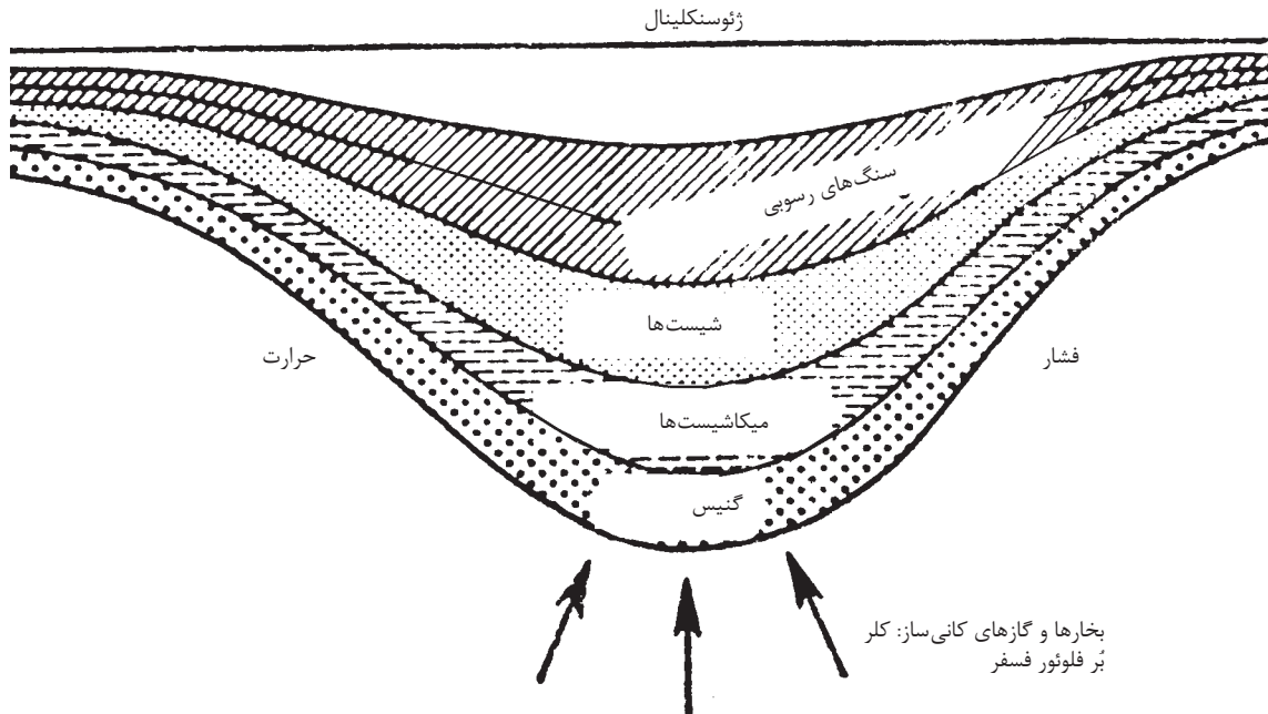
شکل ۲-۵۳- دگرگونی ناحیه‌ای (۴)
