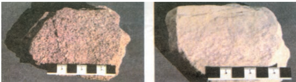
شکل ۲-۴۵- الف (ماسه سنگ کوارتزی، ب) آرکوز (۴)
