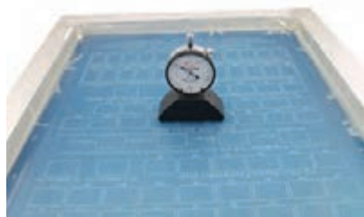
شکل ۵-۲۶ کشش‌سنج توری
