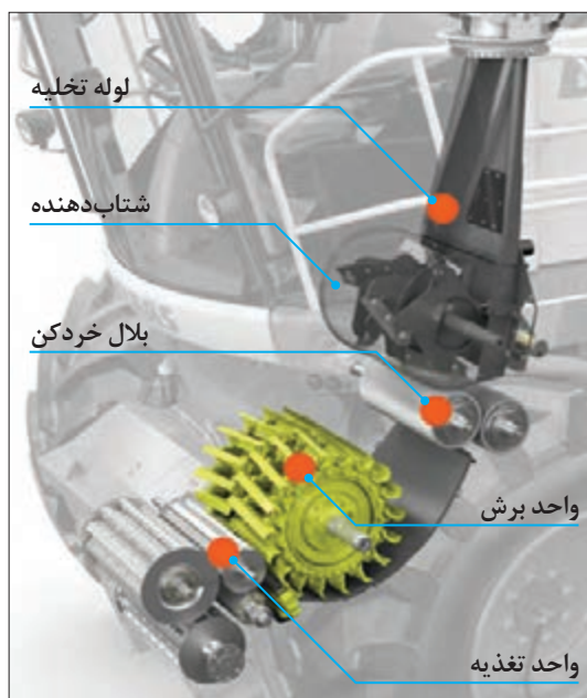
الف) موقعیت واحدها روی ماشین
