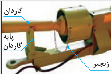
شکل ۵۵- اتصال گاردان به چاپر دو ردیفه
