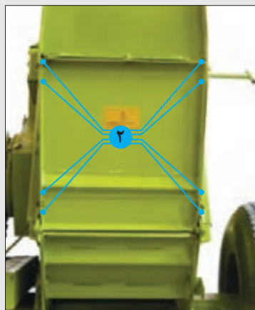
شکل ۶۵- درپوش محافظه برش چاپر دو ردیفه
