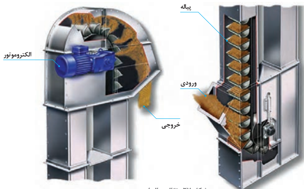
شکل ۲۷- نقاله پیاله‌ای
