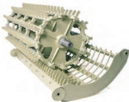
شکل ۱۸- کوبنده و ضد کوبنده چکشی
