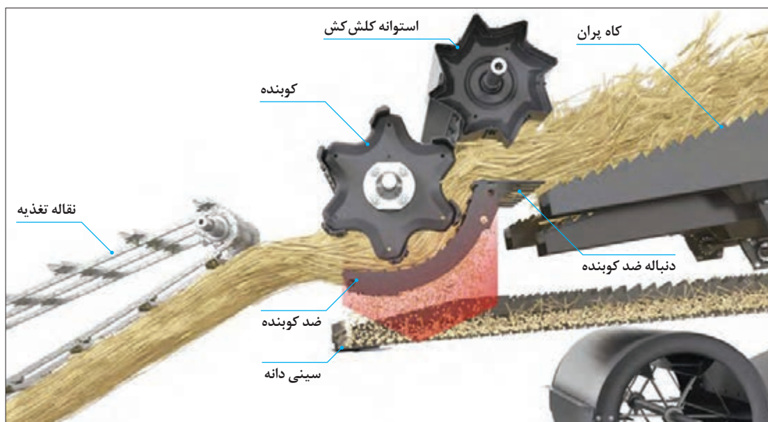
شکل ۱۴- واحد کوبنده
