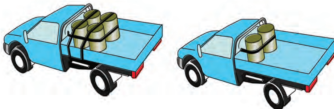
شکل ۳۵- بستن بشکه‌ها توسط بند و استفاده از محافظ‌های کناری و جلویی
