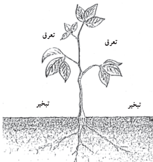
شکل ۱-۱۳- چگونگی تبخیر و تعرق از گیاه و خاک
