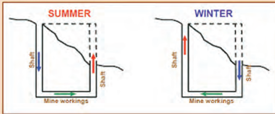
تهویه طبیعی در یک معدن کم عمق و کوچک در فصل‌های زمستان و تابستان
