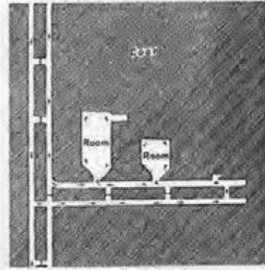
مرحله ۲- شروع استخراج از اتاق‌ها
