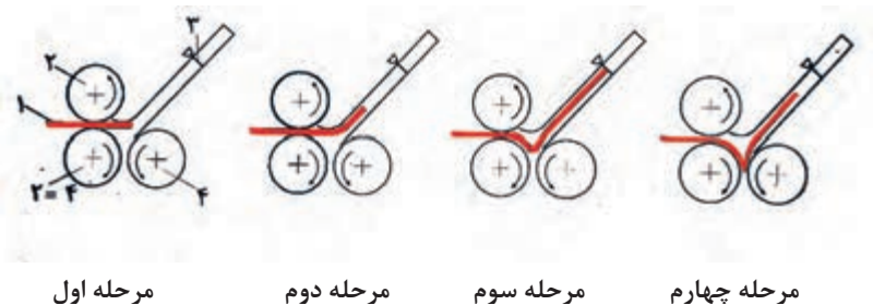
شکل ۶۲- مراحل تای پاکتی
