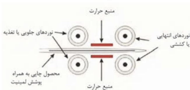
شکل ۴۱- لمینیتور کیسه‌ای یا کتابچه‌ای
