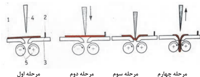
شکل ۶۰- مراحل تای شمشیری
