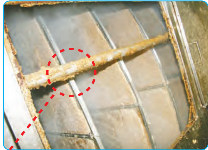
مخزن آهنی برای تولید خمیر کاغذ
