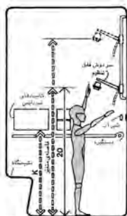
دوش، دسترس پذیری و فواصل مربوط به دوش، ملاحظات انحام سنجی کودکان
