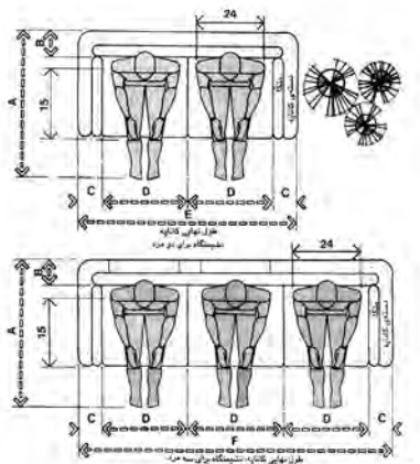
نشیمنگاه کاناپه‌ای، افراد مذکر
