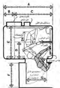
حداقل فواصل مربوط به دوش
