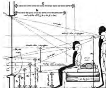
تخت خواب ، دید و خط چشم
