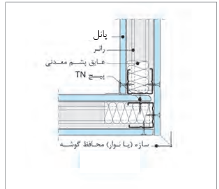
جزئیات پلان از اتصال دو دیوار یک لایه به یکدیگر (اتصال گوشه)
