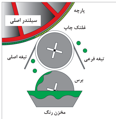
شکل ۱۶- اجزای مهم واحد چاپ گلتنکی
