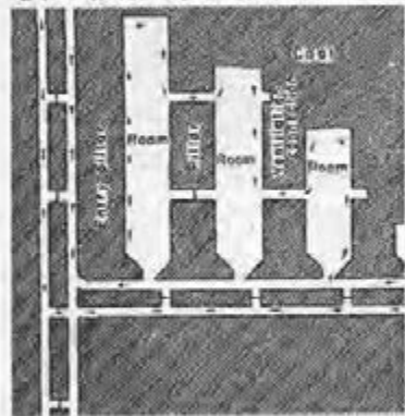
مرحله ۴- استخراج از داخل اتاق‌ها و باقی گذاشتن پایه‌ها
