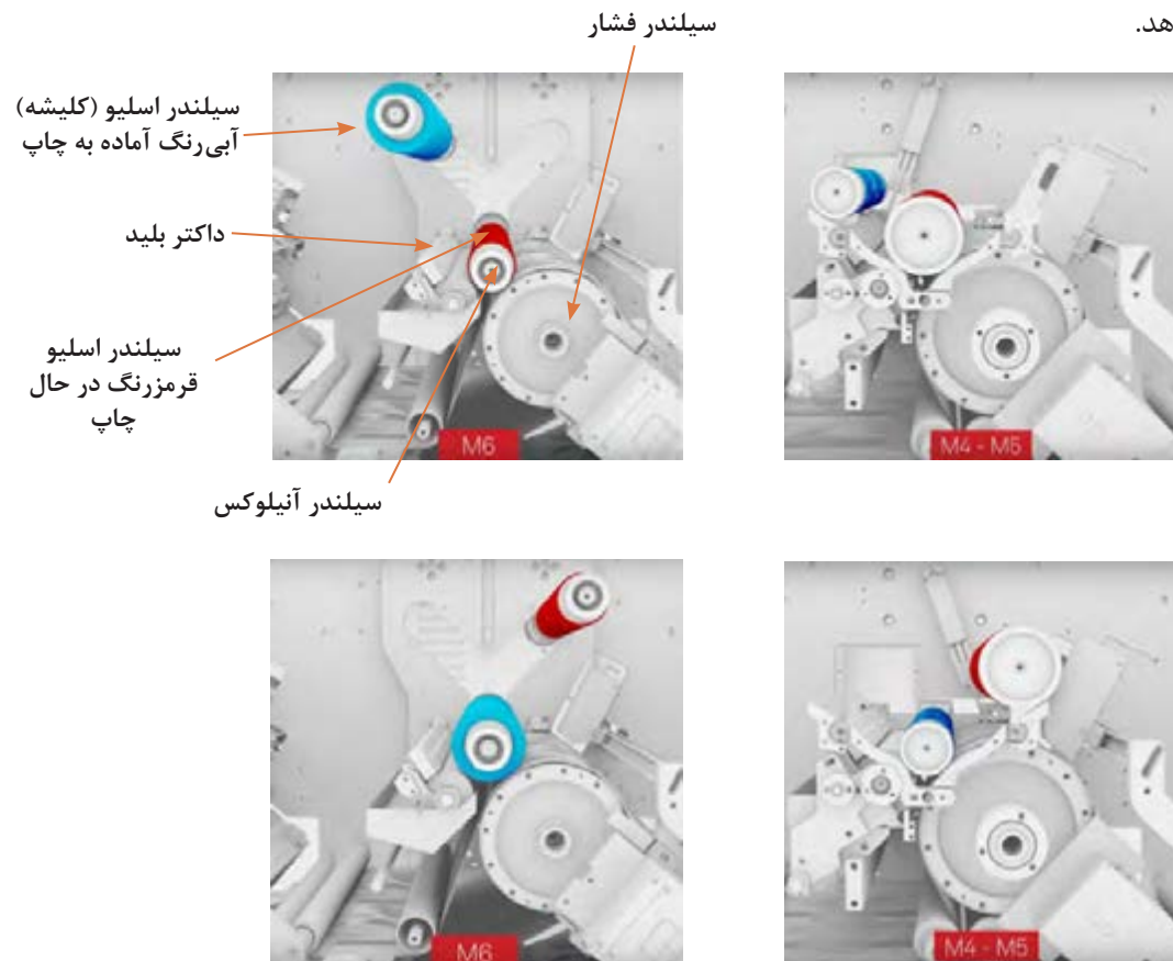
شکل ۳- سیلندر فرم غلافی (اسلیو) در دو ماشین دیجیتال فلکسو
