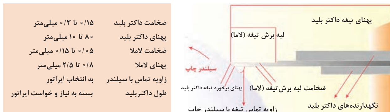
شکل ۷۰- مشخصات داکتر بلید
