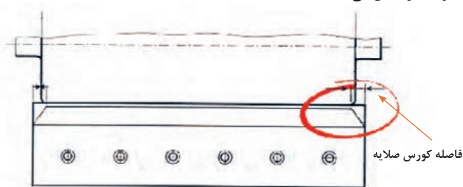
شکل ۷۹- کورس صلیبه تیغه داکتر بلید
