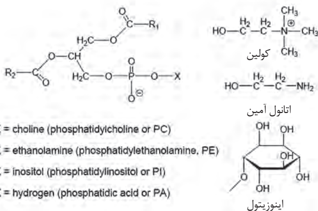
شکل ۲- ساختار شیمیایی فسفاتیدهای عمده در روغنهای گیاهی خوراکی
