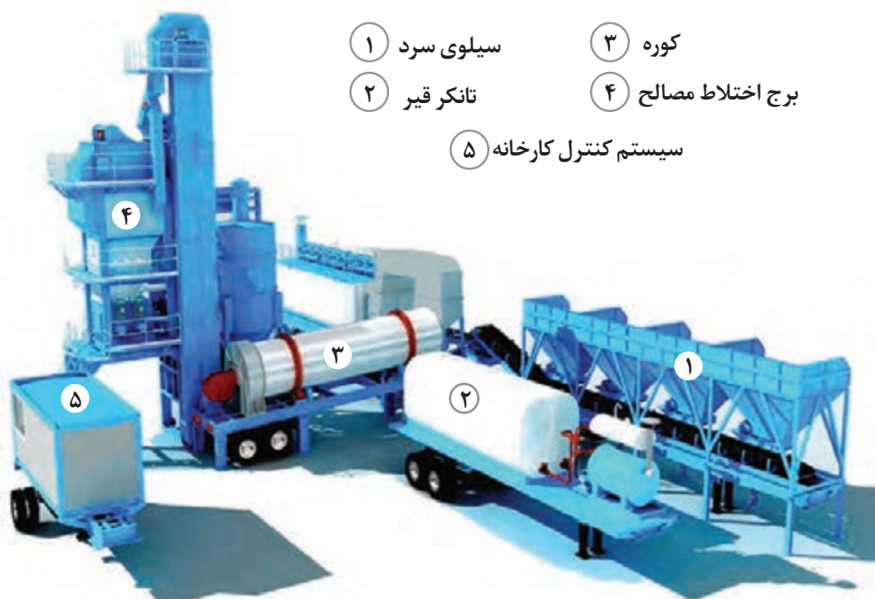
شکل ۳۰- اجزای تشکیل دهنده یک کارخانه آسفالت
