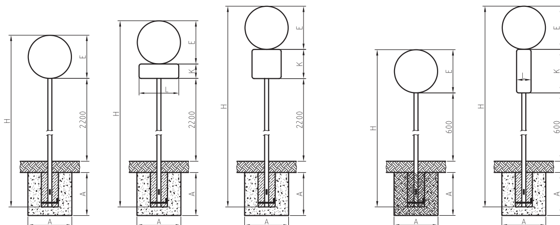
شکل ۶۴- ترکیب نصب‌های متداول تابلوها ابعاد برحسب میلی‌متر
