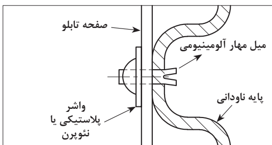
(ب) میل مهارهای آلومینیومی پرچ شونده
