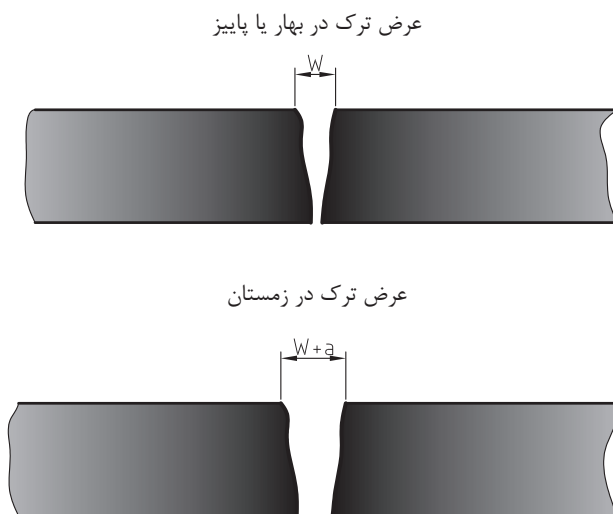
شکل ۱۱- تغییر عرض ترک به واسطه تغییرات دمایی در طول سال
