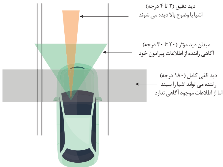
شکل ۱۶- مخروط دید
