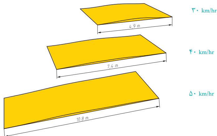
شکل ۲۲- ارتباط عرض سرعت‌گاه و سرعت ترافیک
