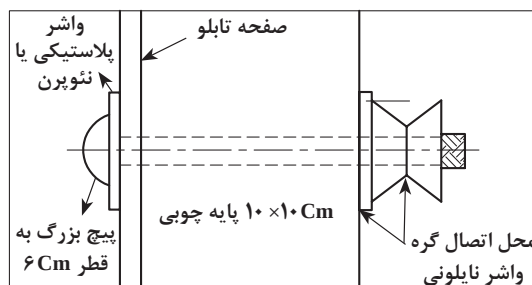
(الف) مهره‌های هرمی شکل
