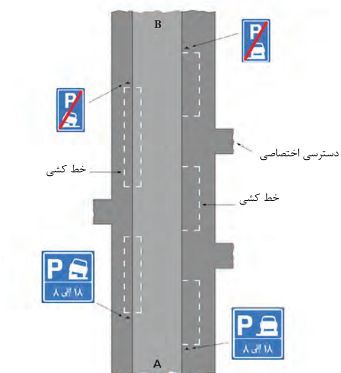
شکل ۳۹ - نمونه‌ای از جانمایی تابلوهای پارکینگ
