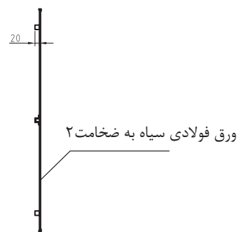
تابلوی مستطیلی به ابعاد ۱۰۰۰×۷۰۰ میلیمتر
