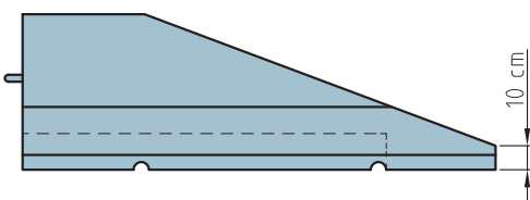
شکل ۷۵- شیب دار کردن انتهای حفاظ های بتنی
