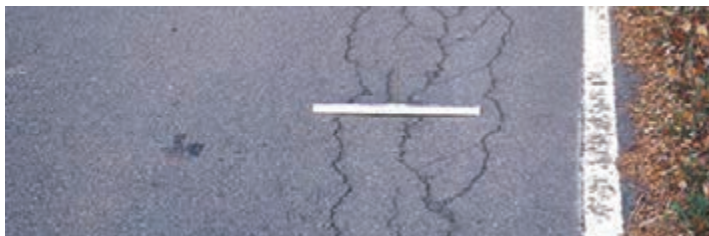
شکل ۳۷- ترک پوست سوسماری در سطح آسفالت
