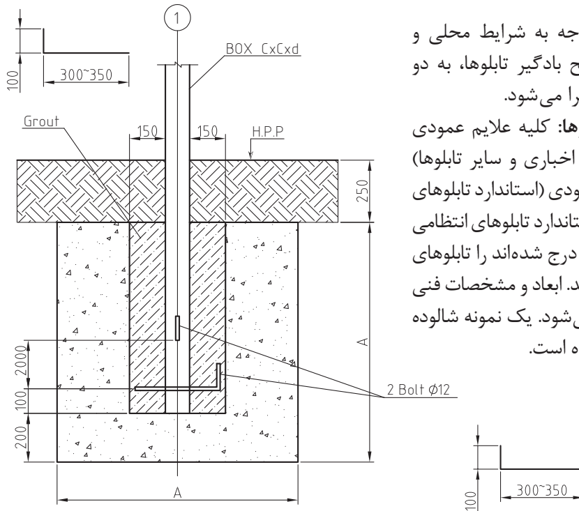
شکل ۵۱ - نقشه اجرایی شالوده تابلوها/ ابعاد برحسب میلی متر (مقطع عرضی)
