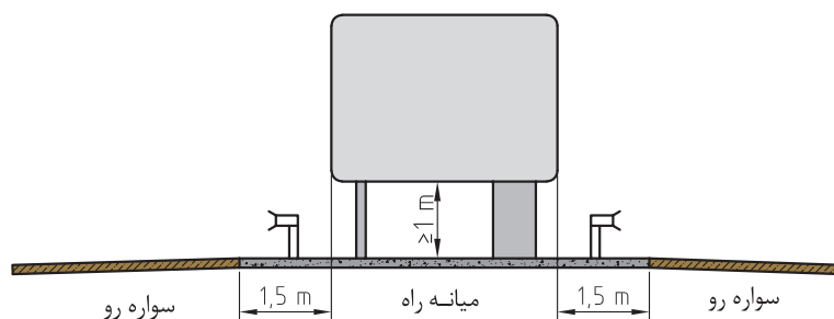
شکل ۵۸ - ارتفاع و فاصله نصب تابلوهای واقع در میانه بزرگراه‌ها
