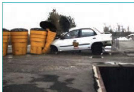
شکل ۱۲- تخریب ضربه گیرهای وزنی بشکه ای بعد از برخورد
