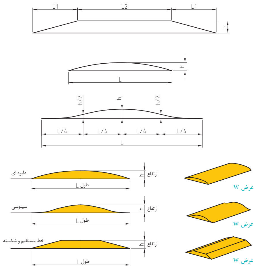
شکل ۲۱- انواع مقاطع عرضی رمپ ورودی سرعت‌گاه‌ها
