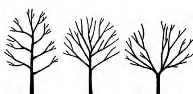
هرس هرمی
