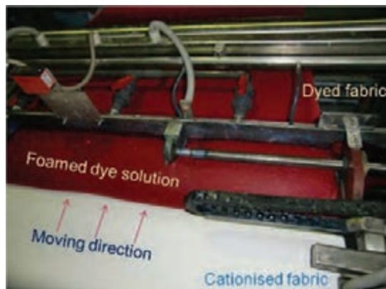
شکل ۱۹- نحوه رنگریزی با کف
