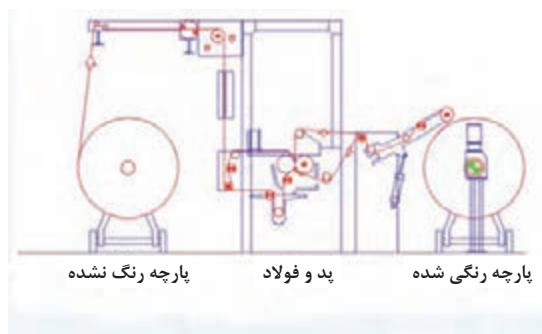
شکل ۲۰- حرکت پارچه در ماشین پد - فولارد
