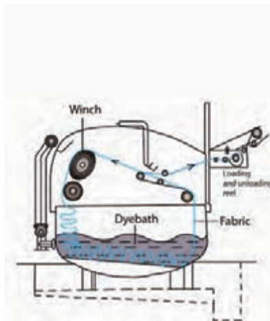
شکل ۱۷- مسیر پارچه در ماشین رنگری وینچ
