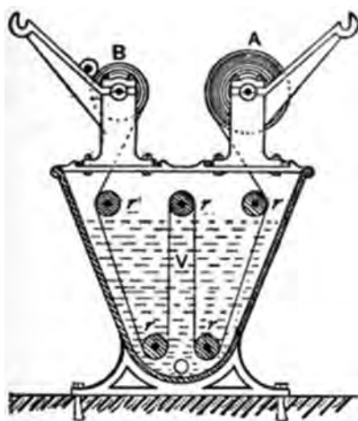
شکل ۱۶- نمای یک ماشین رنگری ژیگر
