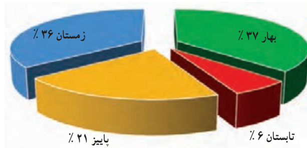
شکل ۱۵- نمودار سهم بارش فصلی استان خراسان شمالی
