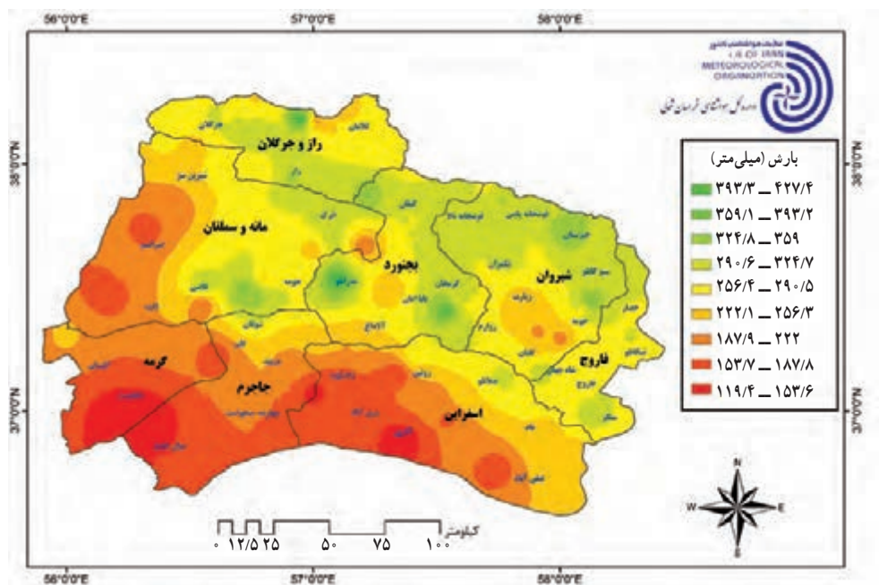
شکل ۱۶- پهنه بندی میانگین بارش سالانه استان خراسان شمالی
