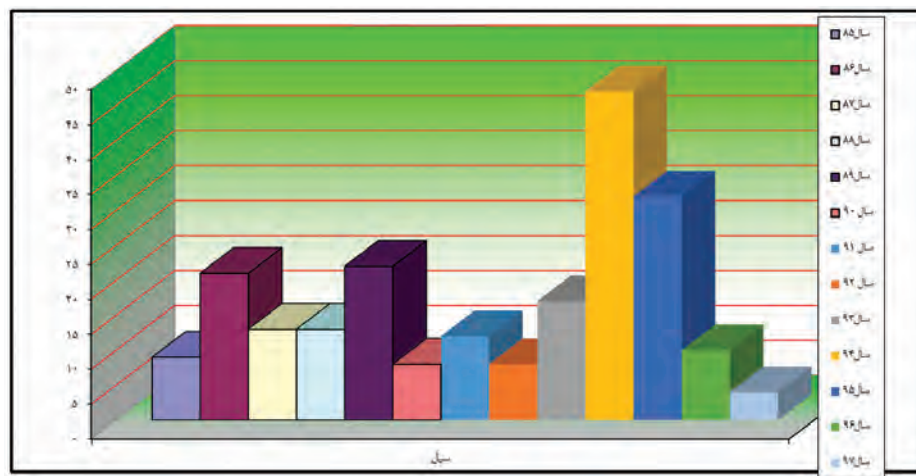
شکل ۷۰-۱- بحران سیلاب سال‌های ۱۳۸۵-۱۳۹۷
