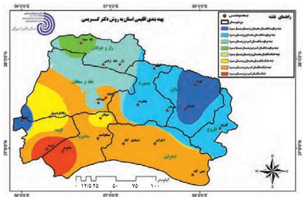
شکل ۱۸-۱- طبقه‌بندی اقلیمی خراسان شمالی با استفاده از روش دکتر کریمی
