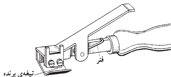
شکل ۵-۲۴- سیم‌چین درآر طولی کابل
