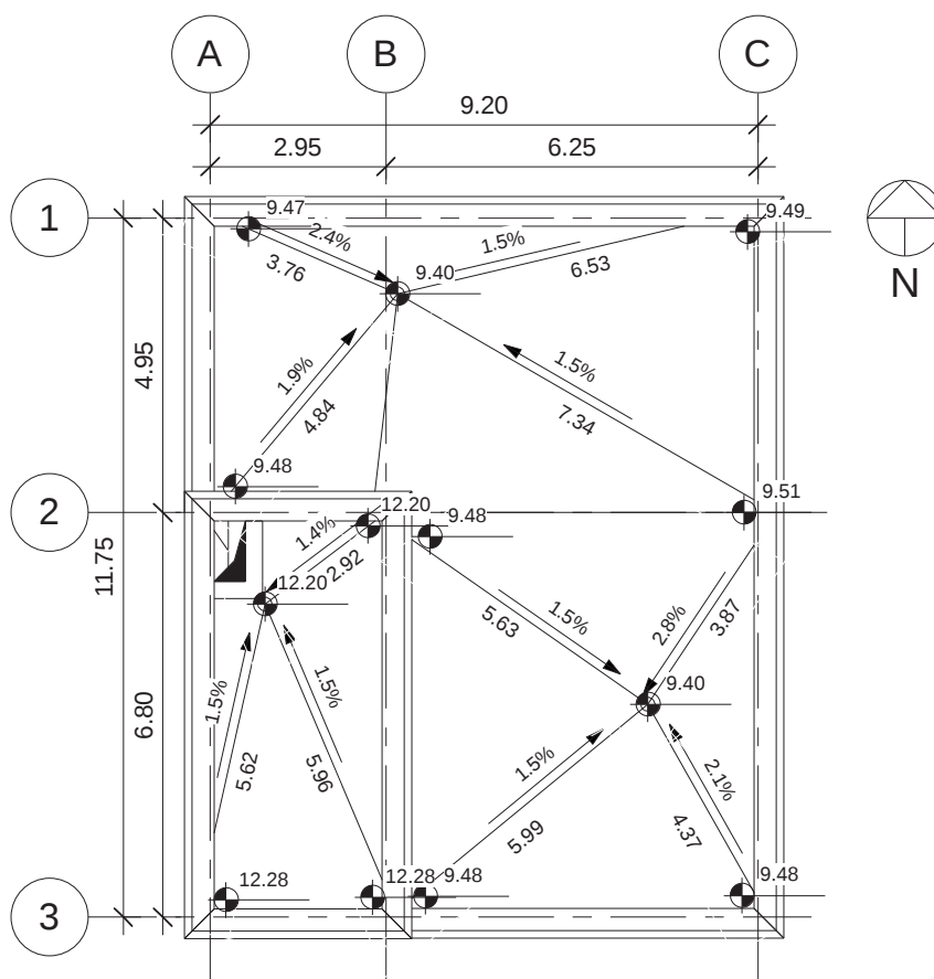
۱ پلان شیب بندی بام
