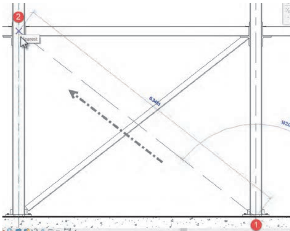
شکل ۶۰ ▲ ترسیم بادبند
